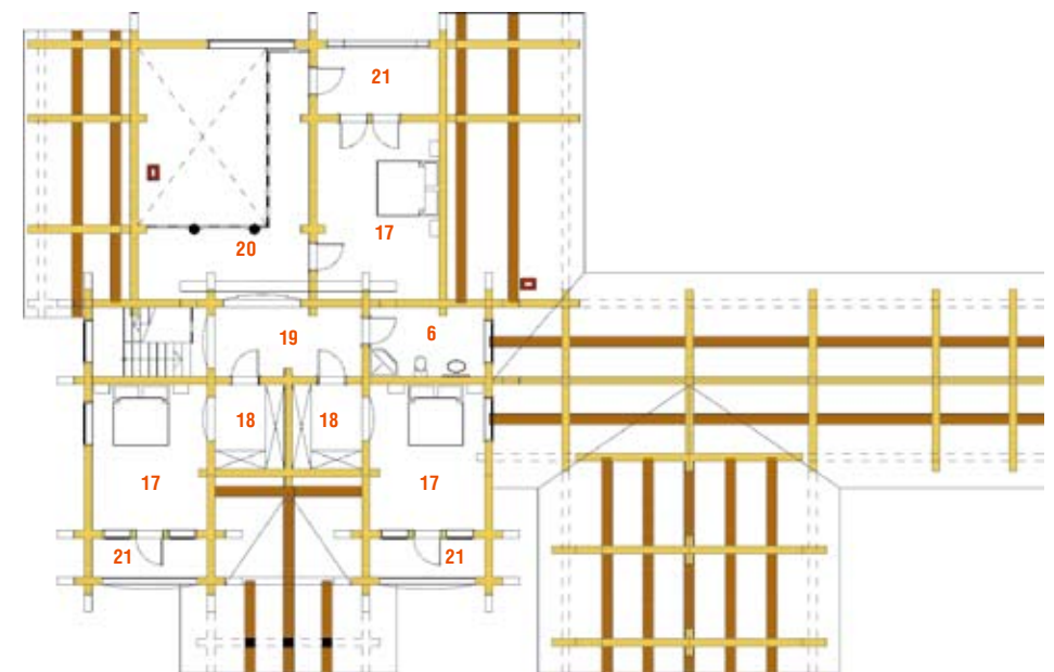
ПЛАН МАНСАРДНОГО ЭТАЖА
